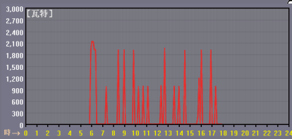
飲水機加裝定時器用電趨勢圖
