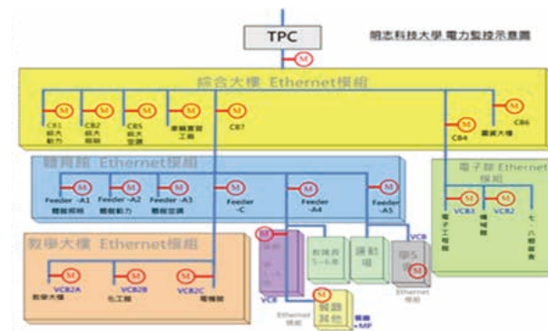
電力監控示意圖
