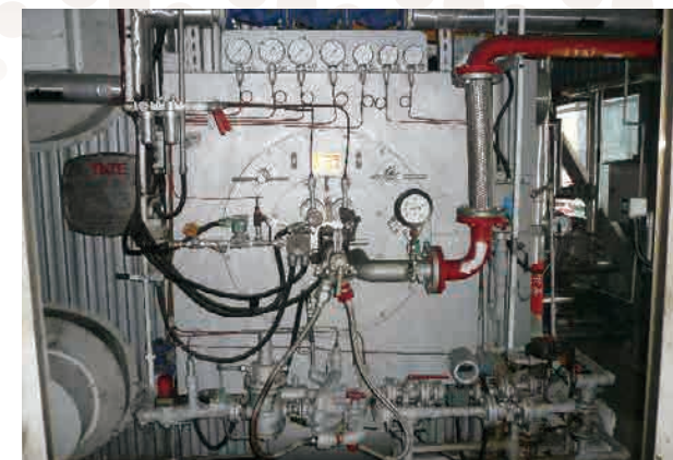
6 噸鍋燃氣系統
