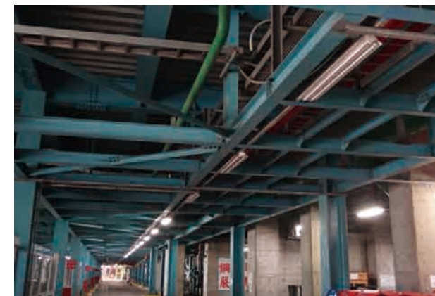
照明燈具改用 T5 燈管
